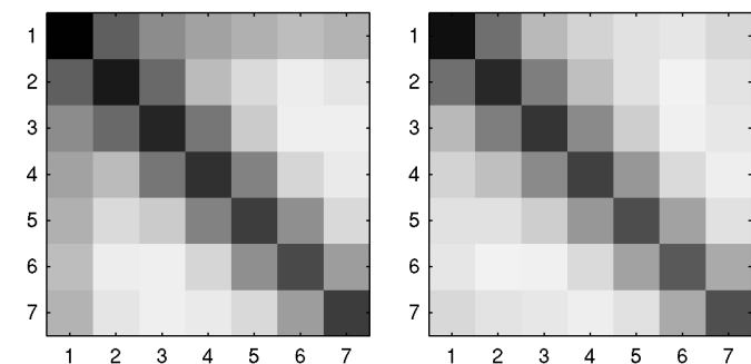
FIG. 4 – Normes des spectres-interspectres moyens des IMFs obtenus avec le deuxième algorithme pour : (a) le bruit blanc simple; (b) le bruit blanc analytique. (codage logarithmique en niveaux de gris, dynamique de 30 dB)
