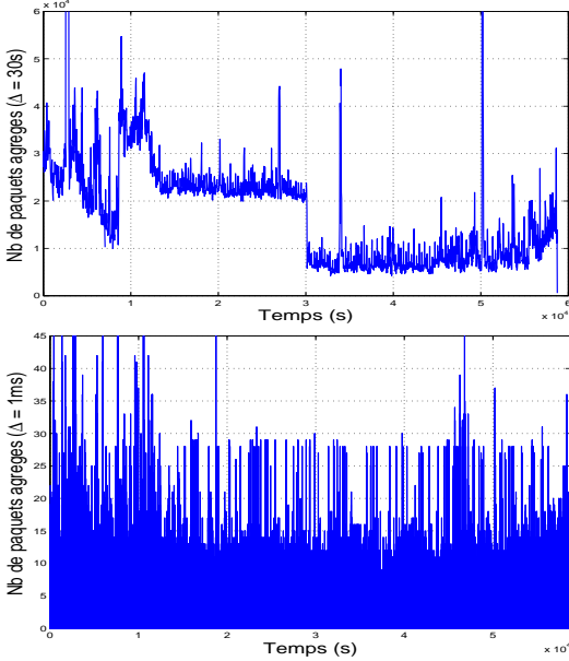
FIG. 1 – Séries temporelles obtenues en agréant le nombre de paquets dans des boîtes temporelles successives de taille \Delta = 30s (haut) ou \Delta = 1ms (bas).
